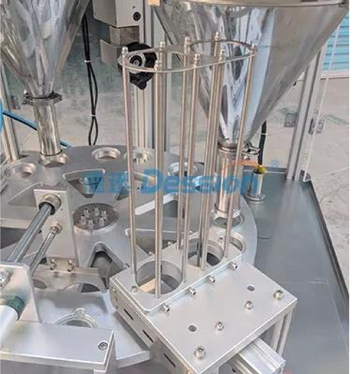
جهاز سقوط الكأس تنزل الكؤوس واحدًا تلو الآخر تلقائيًا.
