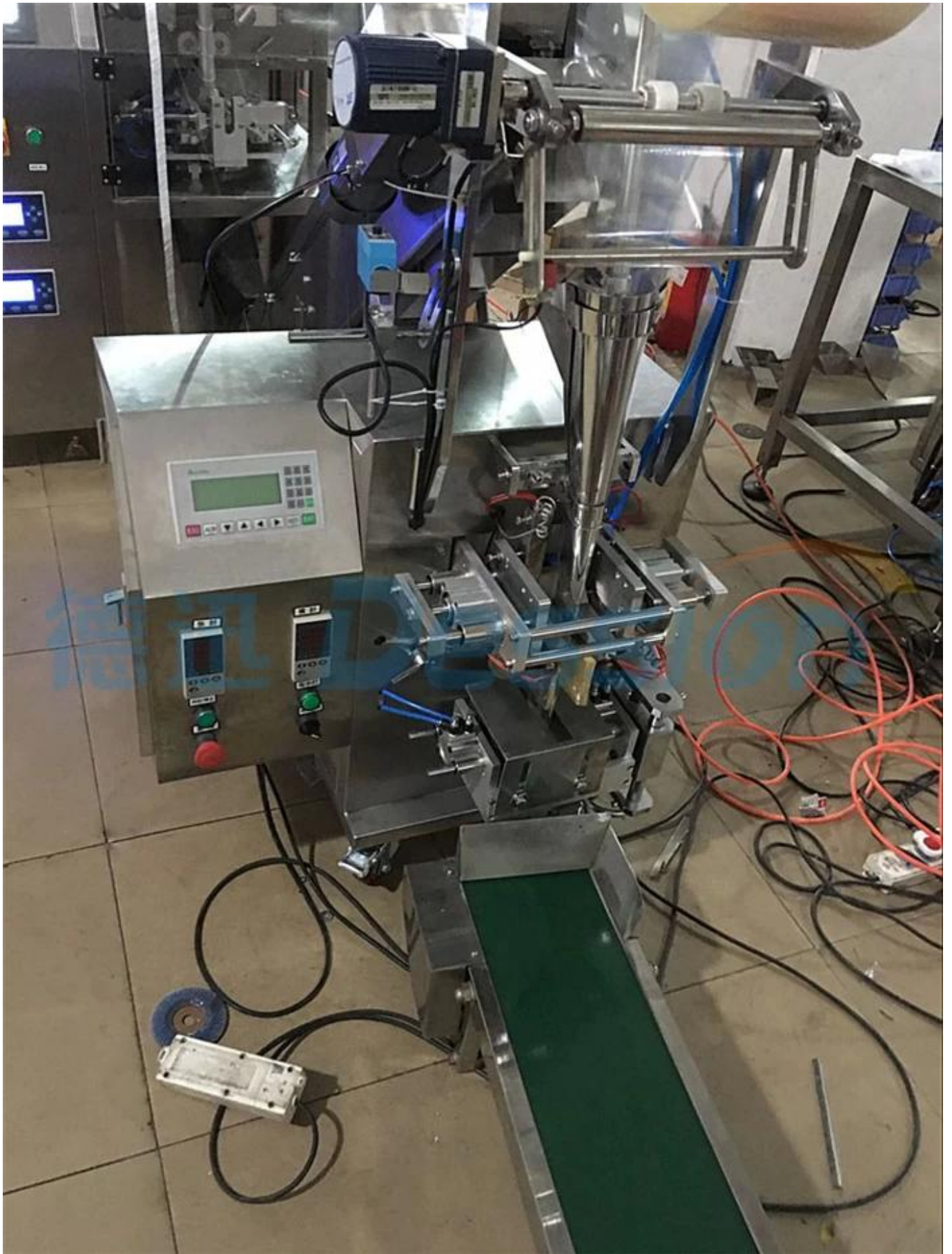
Außenbeutel-Verpackungsmaschine
