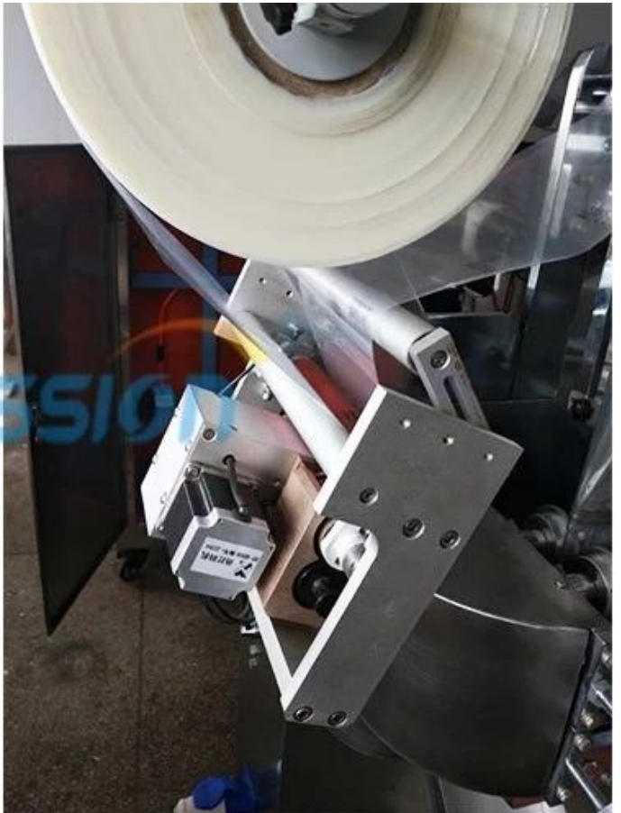
Volumetrisch Tasse Messung Film Rollen & Position Sensor
