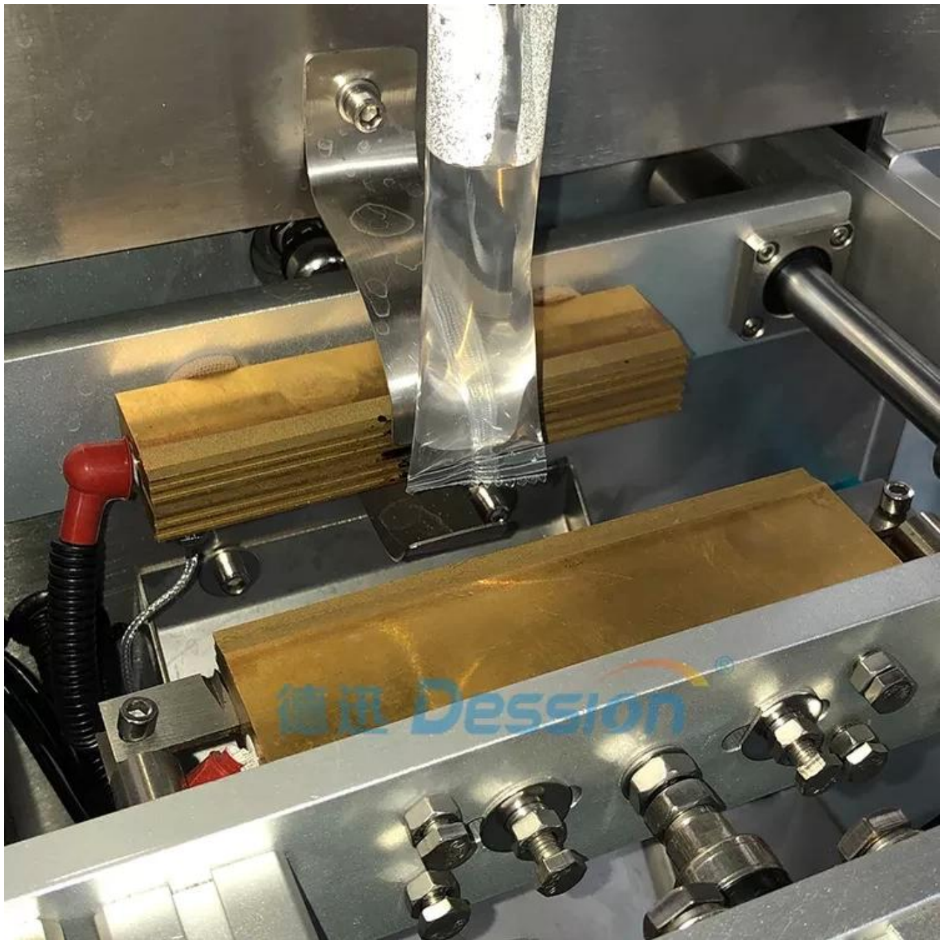
Beutelschneidegerät
