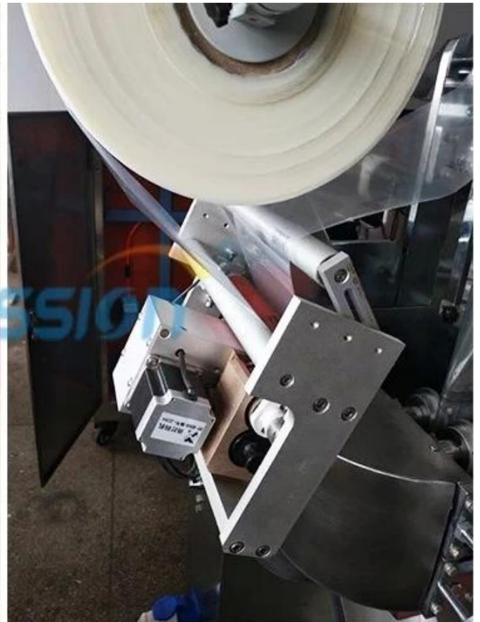
Volumetrisch Tasse Messung Film Rollen & Position Sensor
