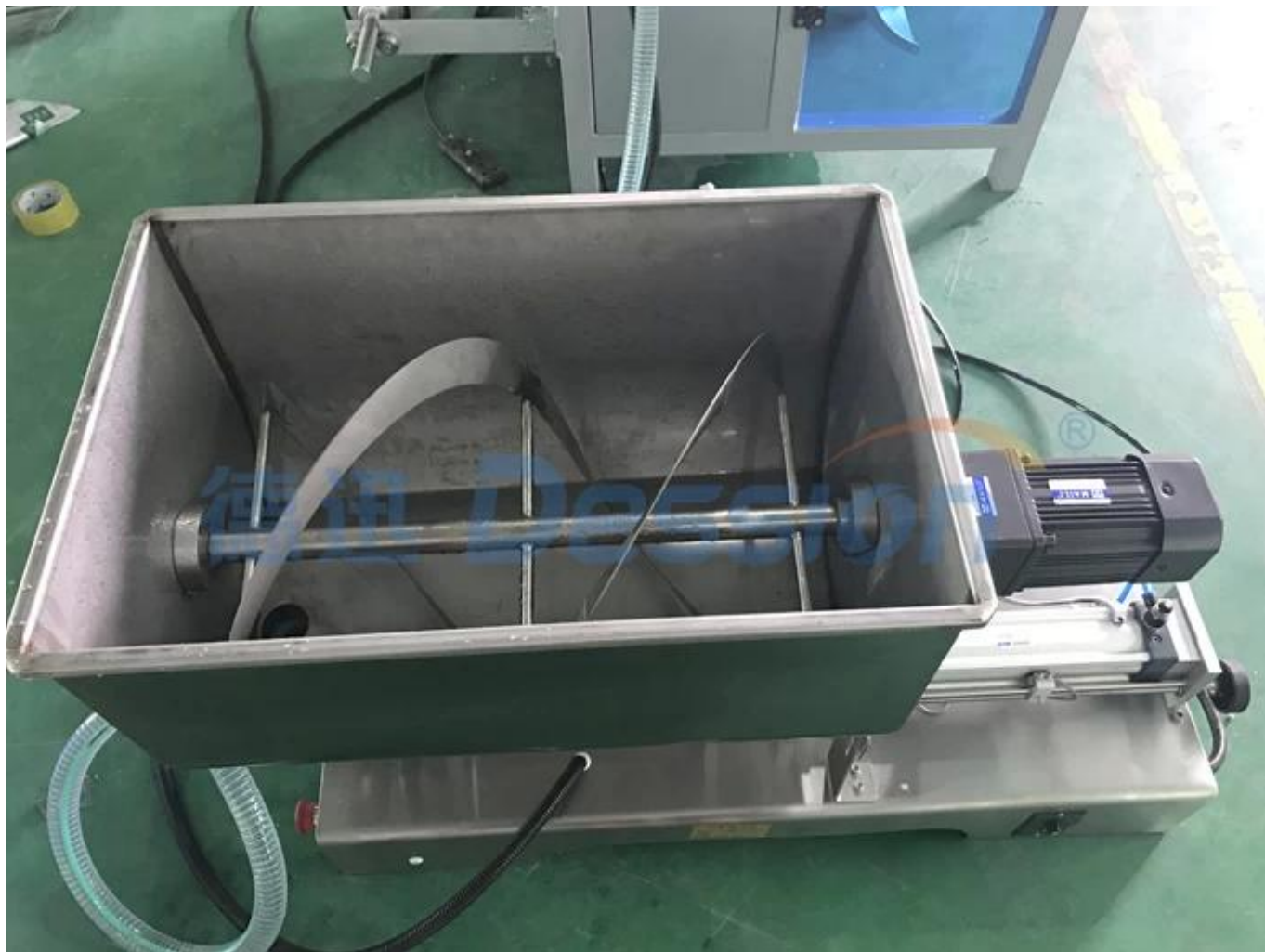
Rührgerät
