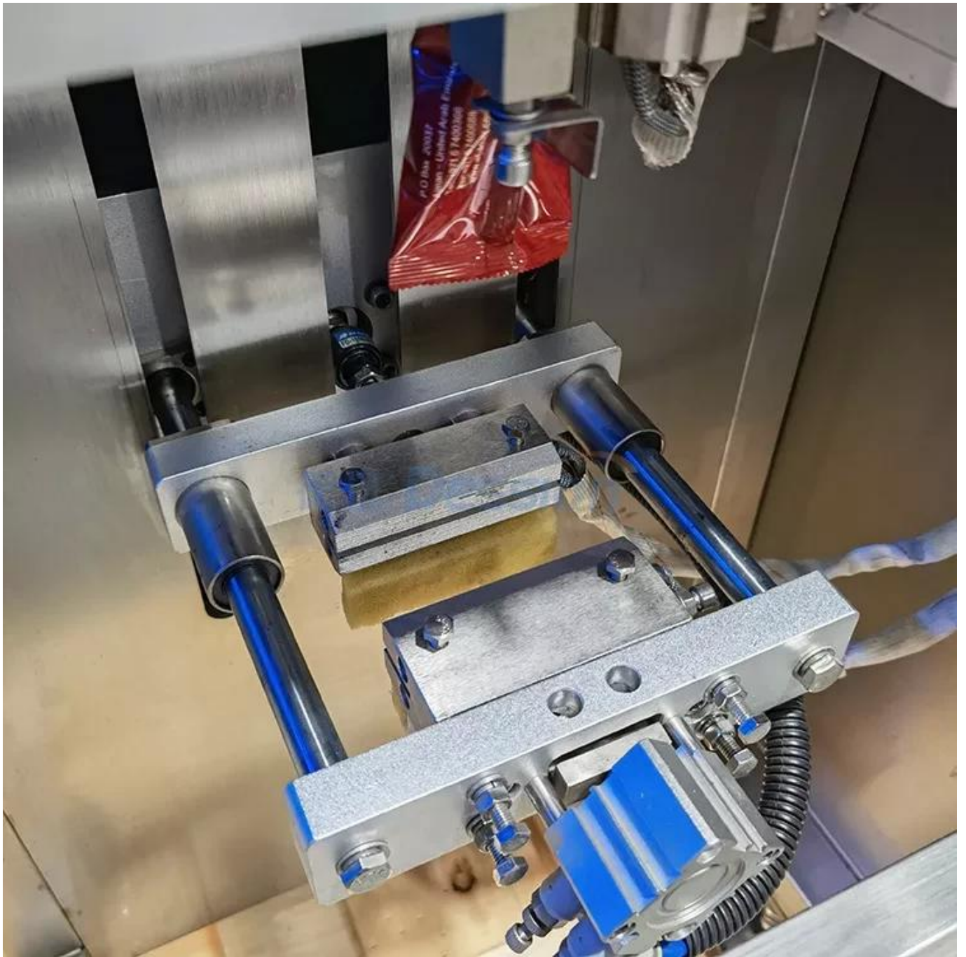
Schneidgerät
