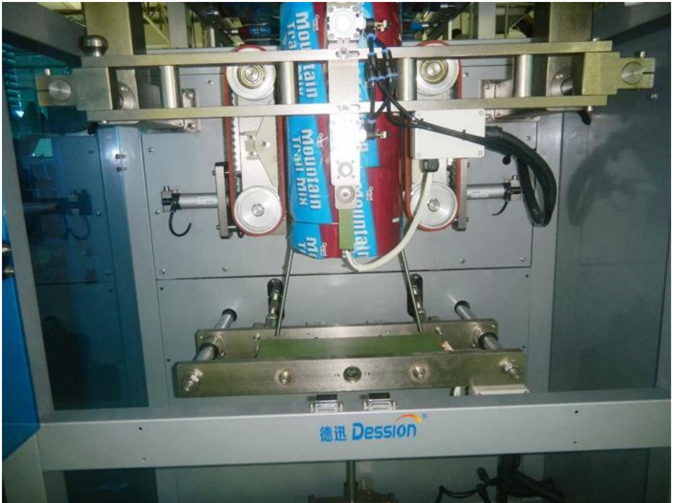
Cuchillo de corte
