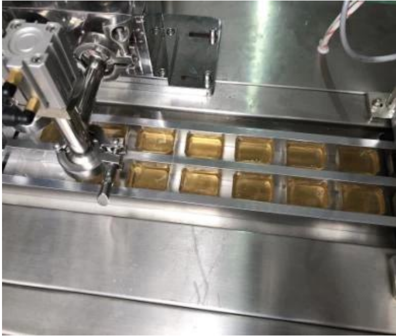
dispositivo de embalaje
