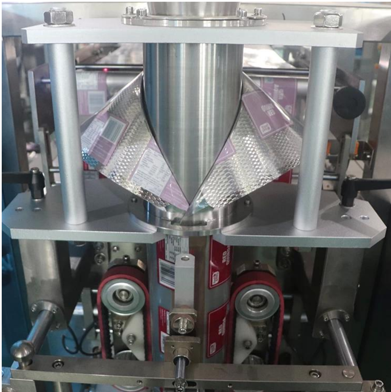
6) Eindsealing bar seal de zak
