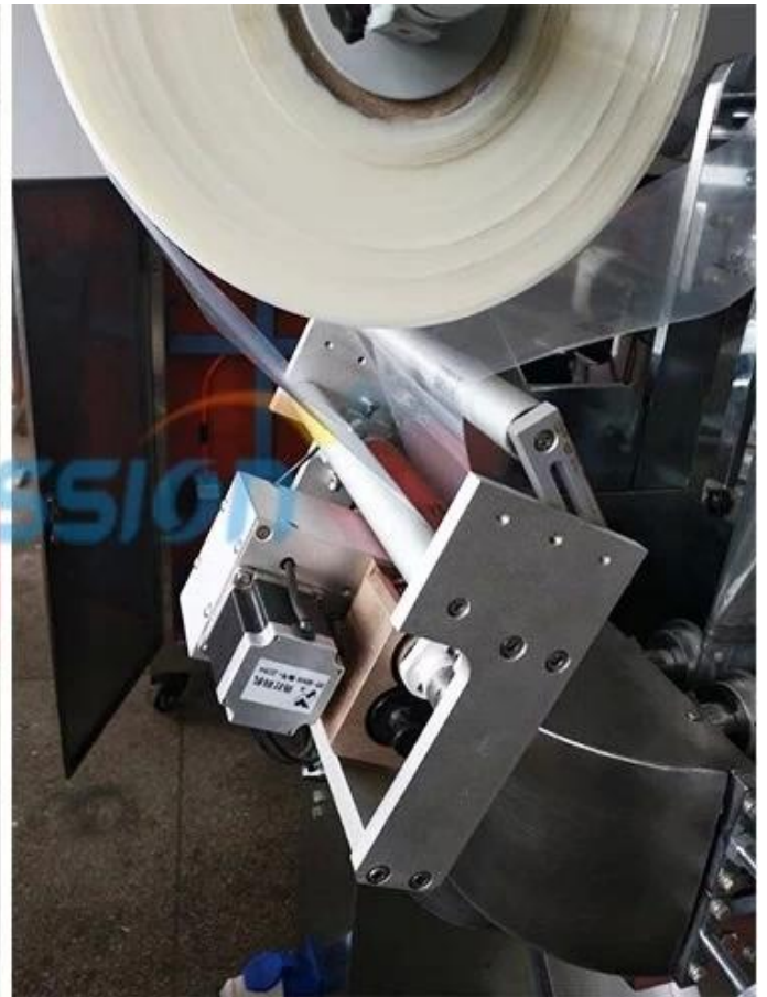
Volumetrisch Beker Meten Film Rollen & Positie Sensor
