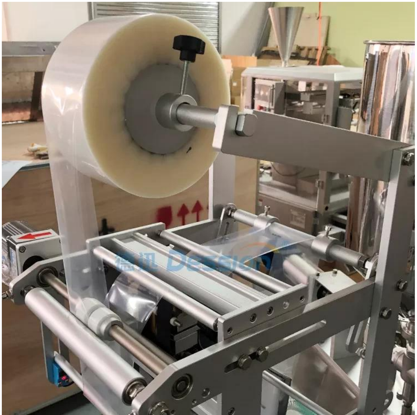
Filmhouder
