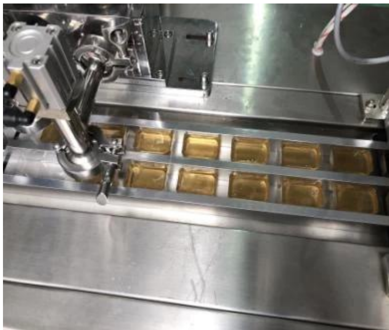
упаковочное устройство
