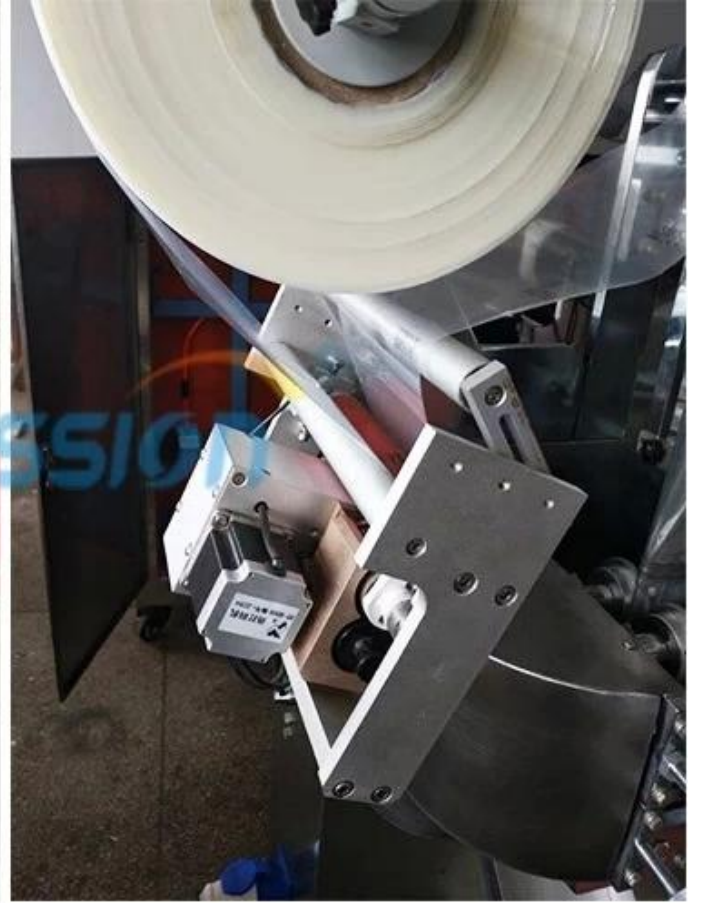
Volumetrik Bardak Ölçüm Film Rulo & Konum Sensör
