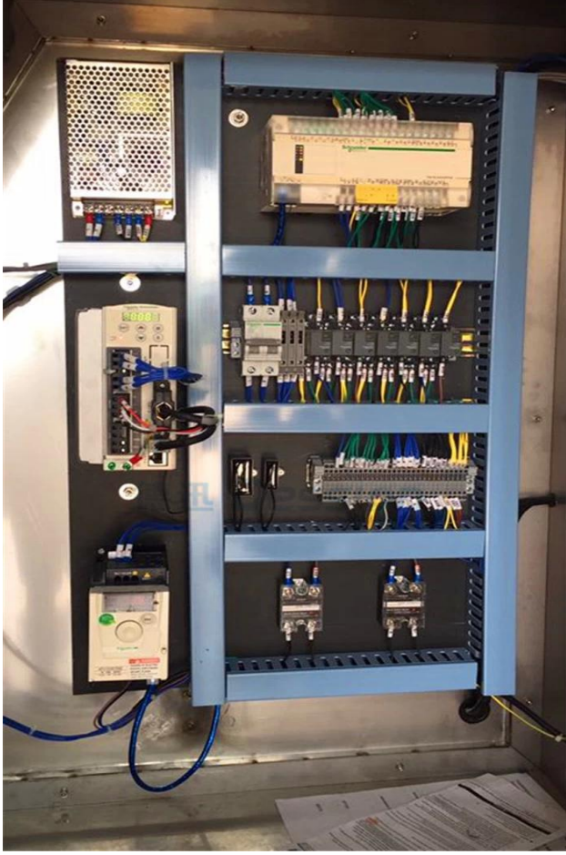
PLC kontrol cihazı
