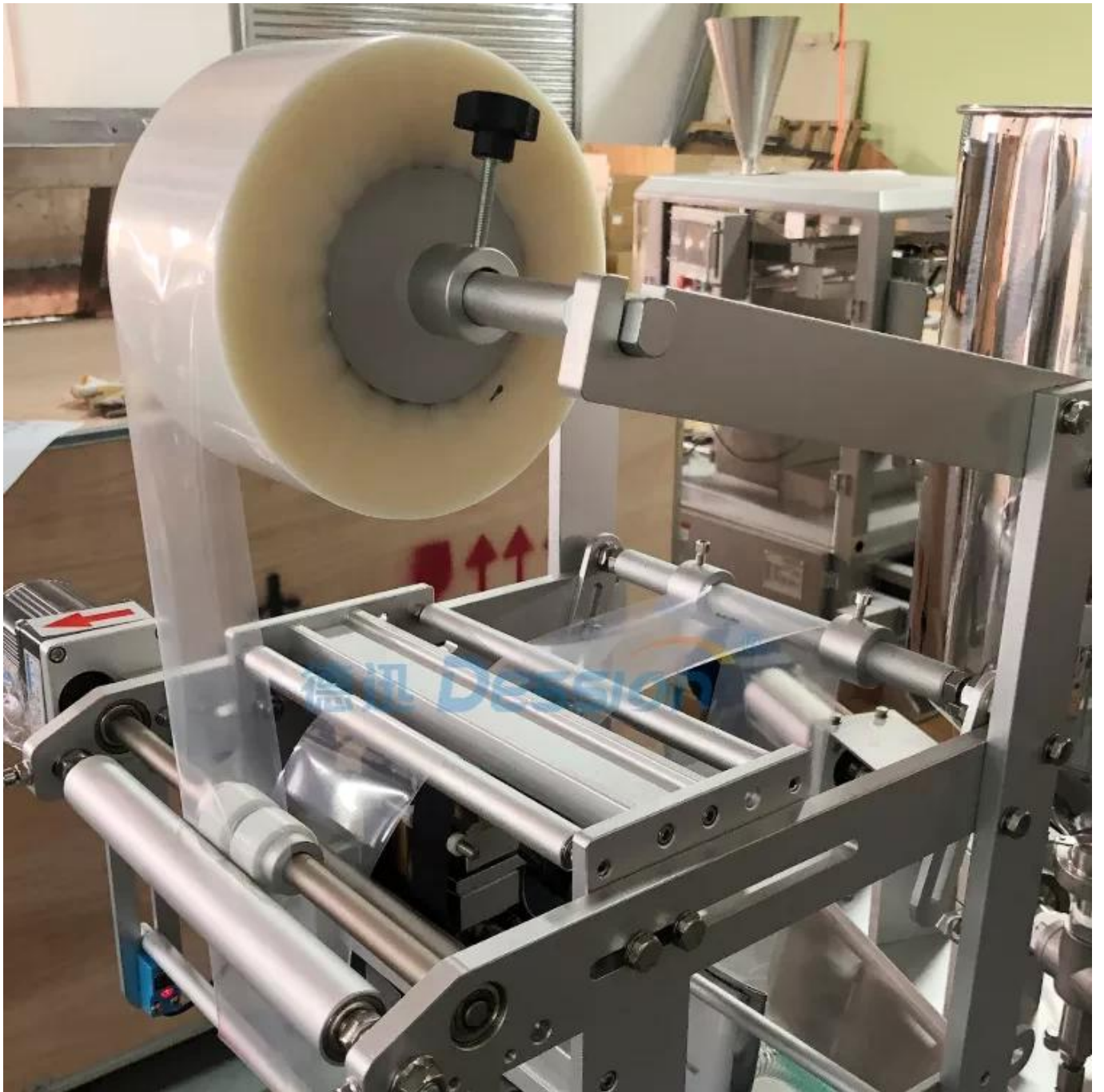
Film Tutucu
